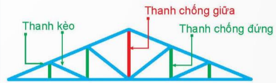
Đây là dạng một vì kèo.
