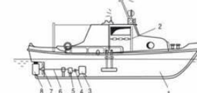
Hình 35.1. Bố trí động cơ và hệ thống truyền lực trên tàu thủy
